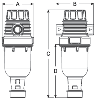
Dimensioni mm
